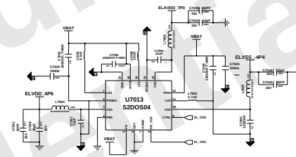
HD OCTA DC-DC
