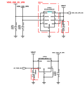
OIS AF LDO
